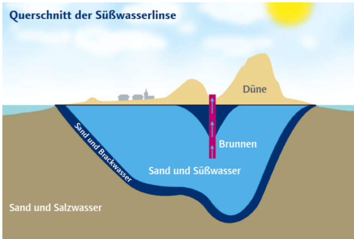
Schematische Darstellung der Süßwasserlinse
